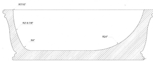
BATH TUB LONGITUDINAL SECTION
